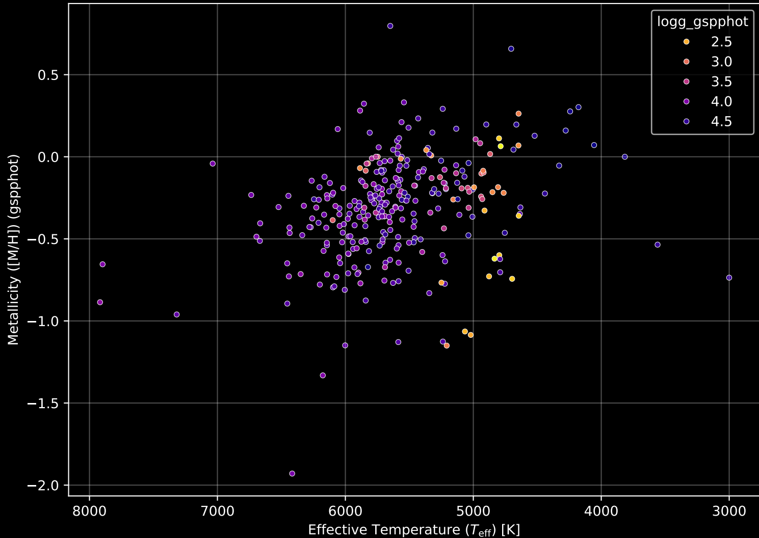
GALAH DR4 Field: [263] Stellar Population Parameters (n= 298)
