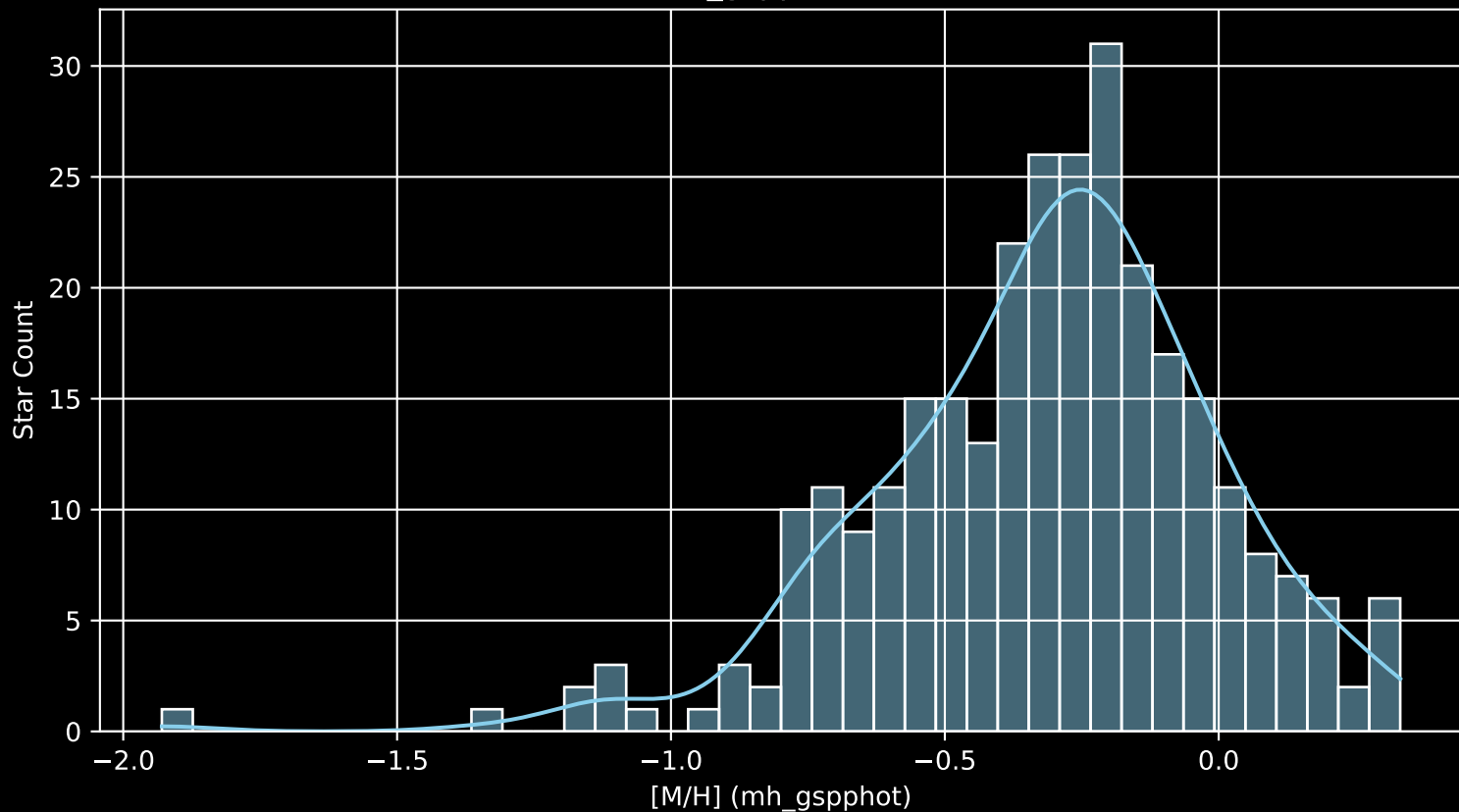
GALAH DR4 Field: [263] [M/H] (mh_gspphot) (n= 296)
