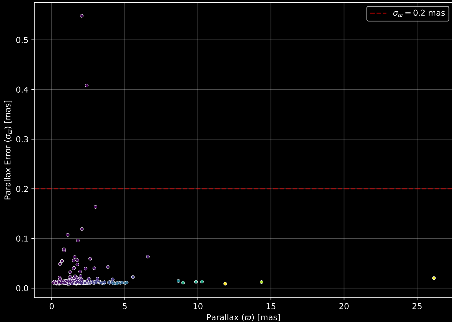
GALAH DR4 Field: [263] Parallax Quality (n= 298)
